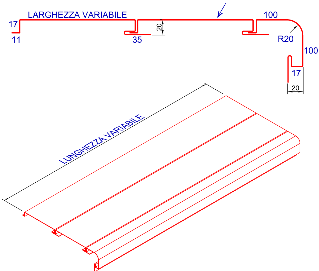
DOGA TECNICA PARTICOLARE IN ALLUMINIO PREVERNICIATO PIEGATO REALIZZABILE CON LARGHEZZA E LUNGHEZZA VARIABILI
