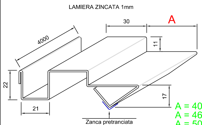
CONTROTELAIO SENZA GUIDA INVERSO
