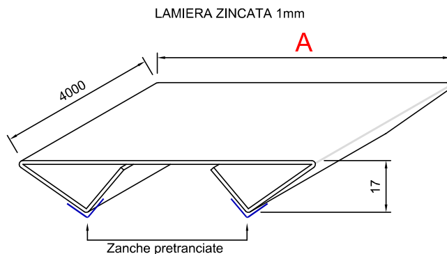
CONTROTELAIO CON GUIDA
